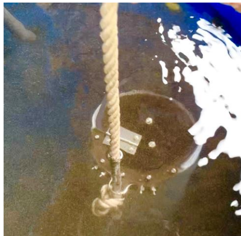
200リットル水槽試験：低層堆積物汲み上げ確認
