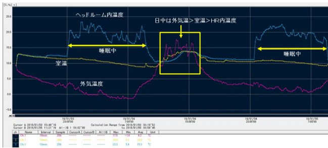
図 29 周辺との温度比較
