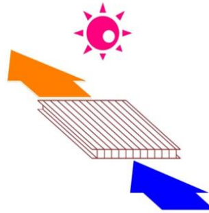
図2 中空ハモニカ構造における採熱原理
