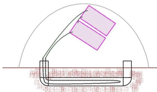
図 20 冬季はパイプ内の水経由での土壌蓄熱
