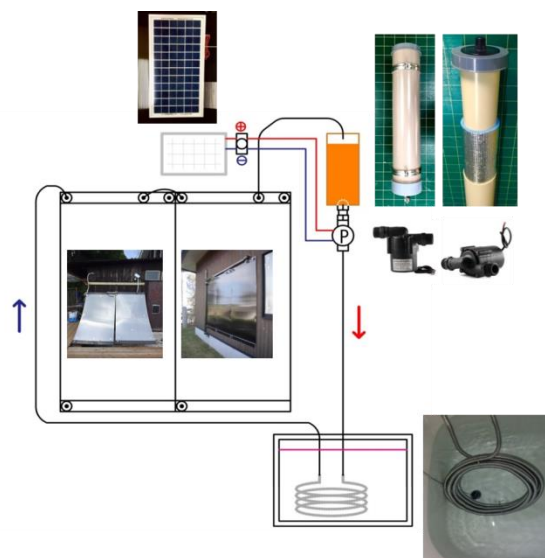
図 7 太陽熱温水システム構成と写真
