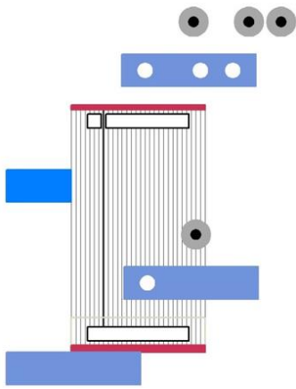
図3 パーツと組み合わせ 部品は右斜め上から左下にかけて 耐熱ノズル、耐熱止水板(表面)、中空ポリカ受光板(上 下の赤色部はシリコン材)、耐熱止水板(裏面)
